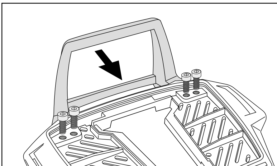
Verlängerung/extension
