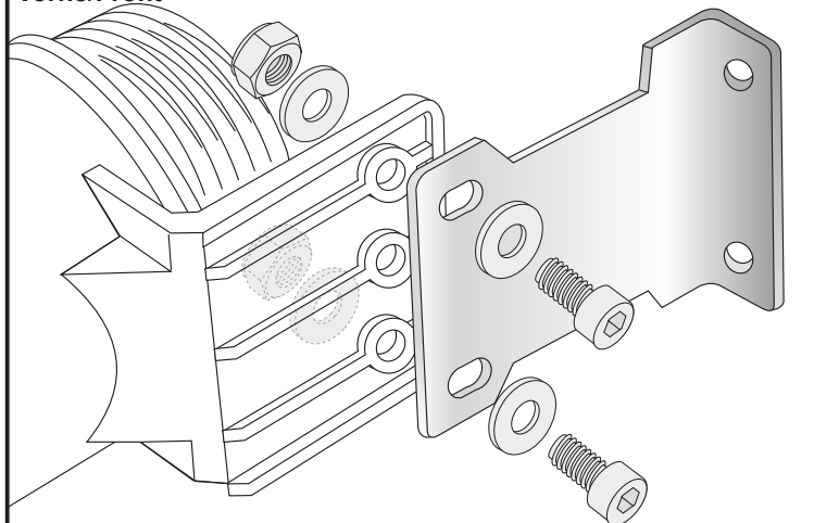
Vorne/Front
